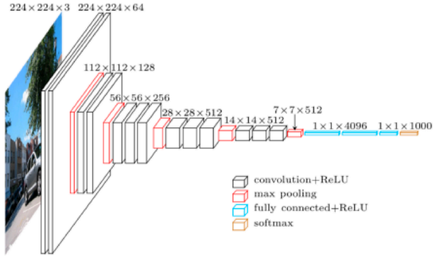
Figure 9. – Réseau de neurones convolutif
