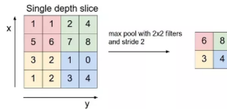
Figure 12. – Représentation du maxpool
