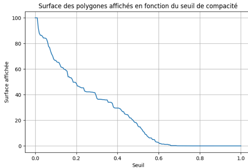
Figure 24. – Evolution de la surface représentée en fonction du seuil choisi
