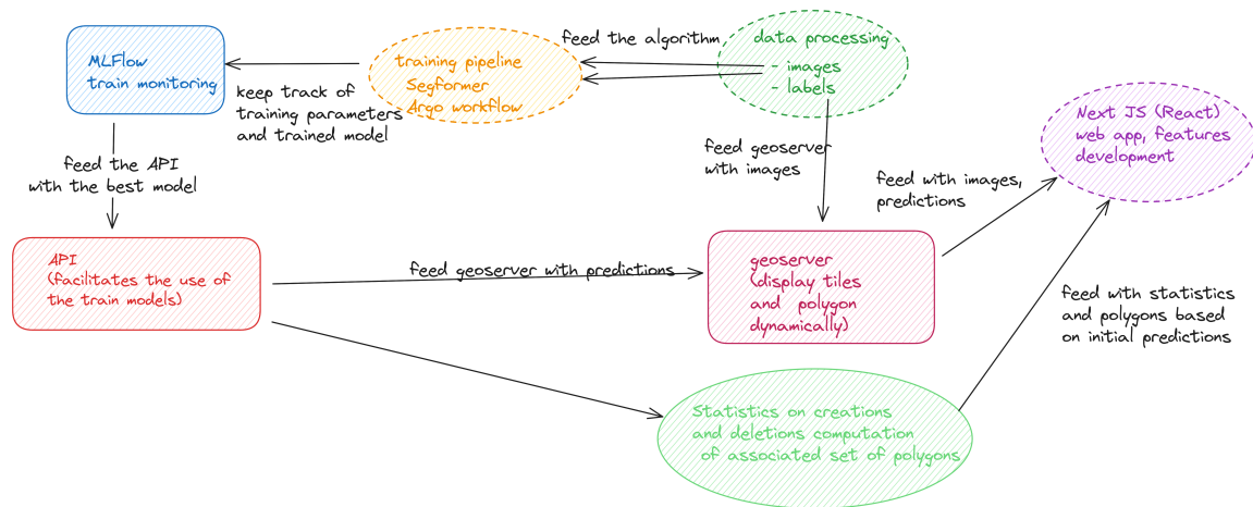
Figure 29. – Représentation schématique de l'ensemble des éléments nécessaires à l'obtention du produit d'aide à la décision assisté par les prédictions de l'algorithme
