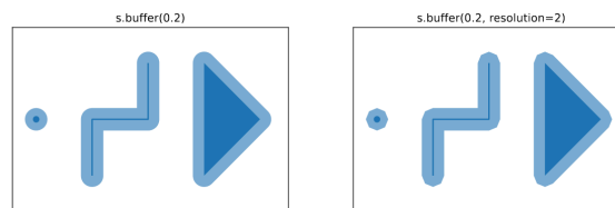
Figure 21. – Exemple de buffer avec deux différentes résolutions
