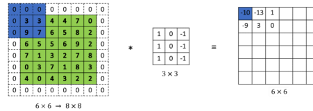
Figure 13. – Représentation du padding
