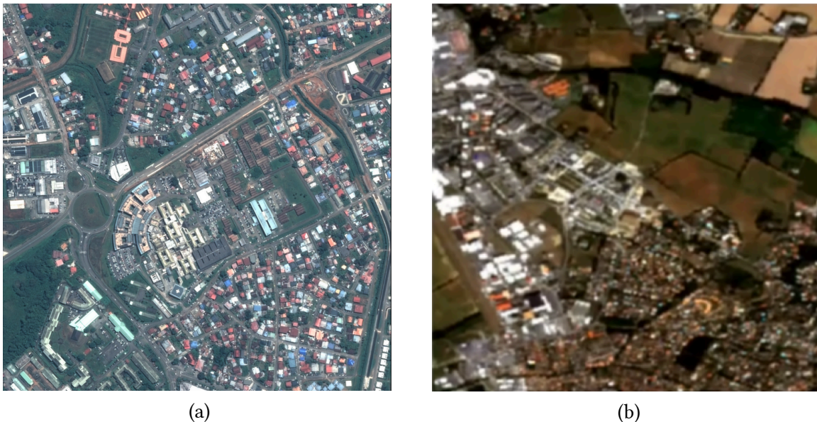
Figure 3. – Comparaison entre une image PLEIADES très haute résolution (a) et une image Sentinel 2 haute résolution (b)
